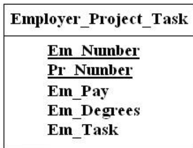
Рисунок 1.15 – ER-діаграма відношення Employer_Project_Task
